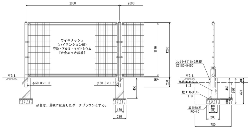
正面図
