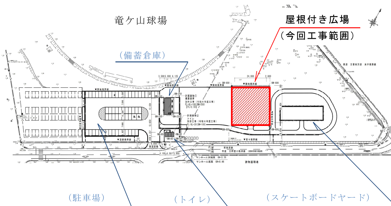
配置図
