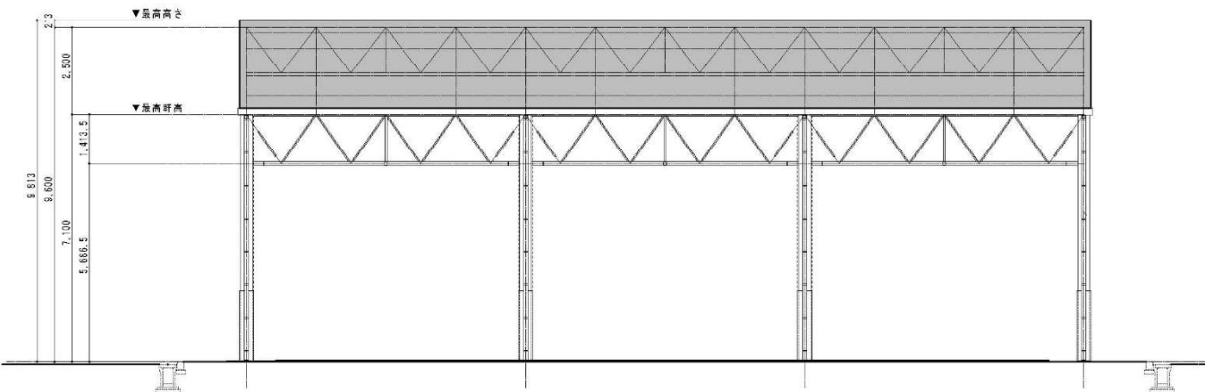
立面图（南側）
