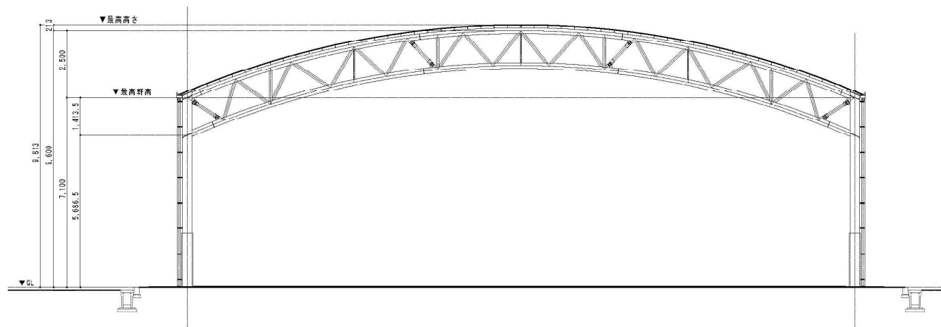
立面图（東側）
