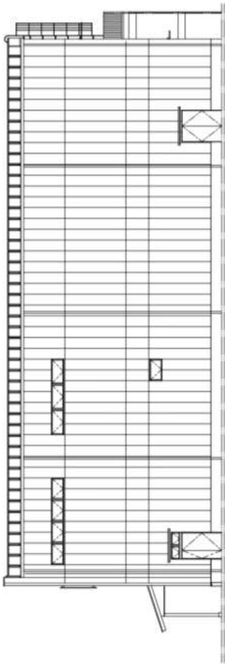
東側立面图
