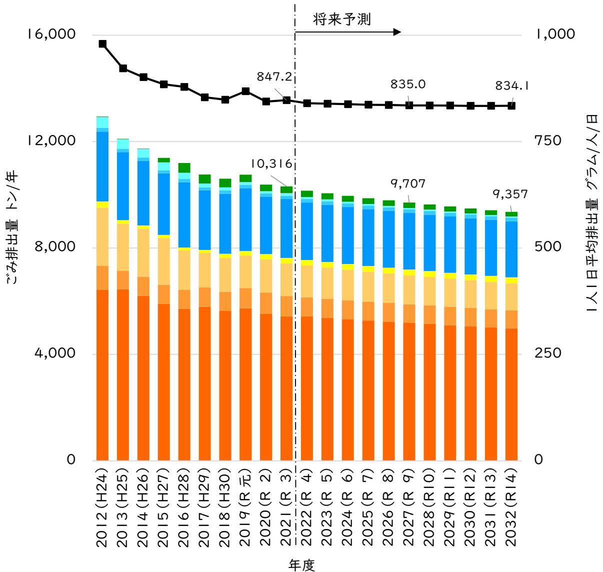
図3-16 ごみ排出量の将来予測（単純推計）
