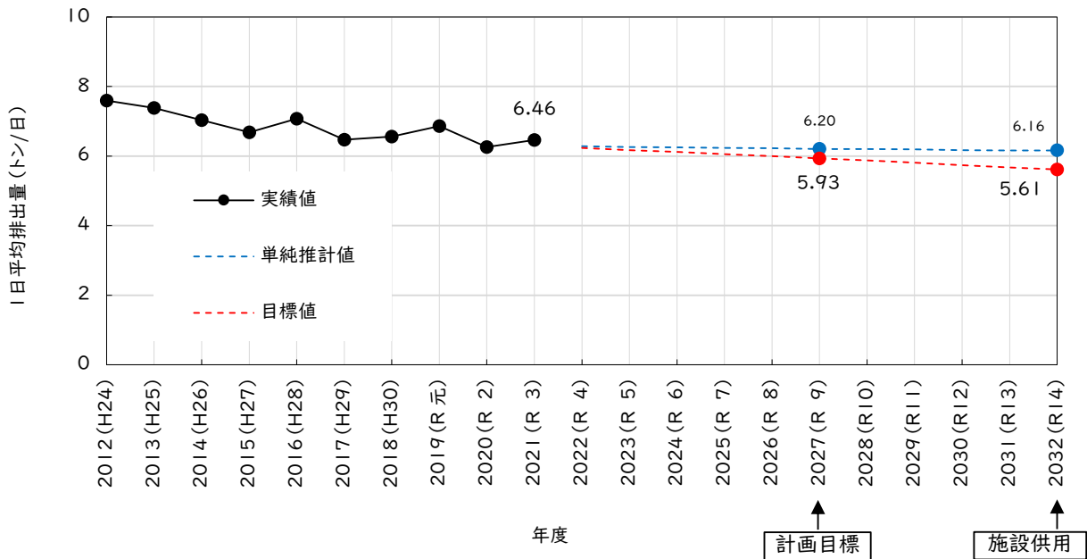
図3-21 事業系ごみ排出量(資源ごみ量除く)の将来見込み
