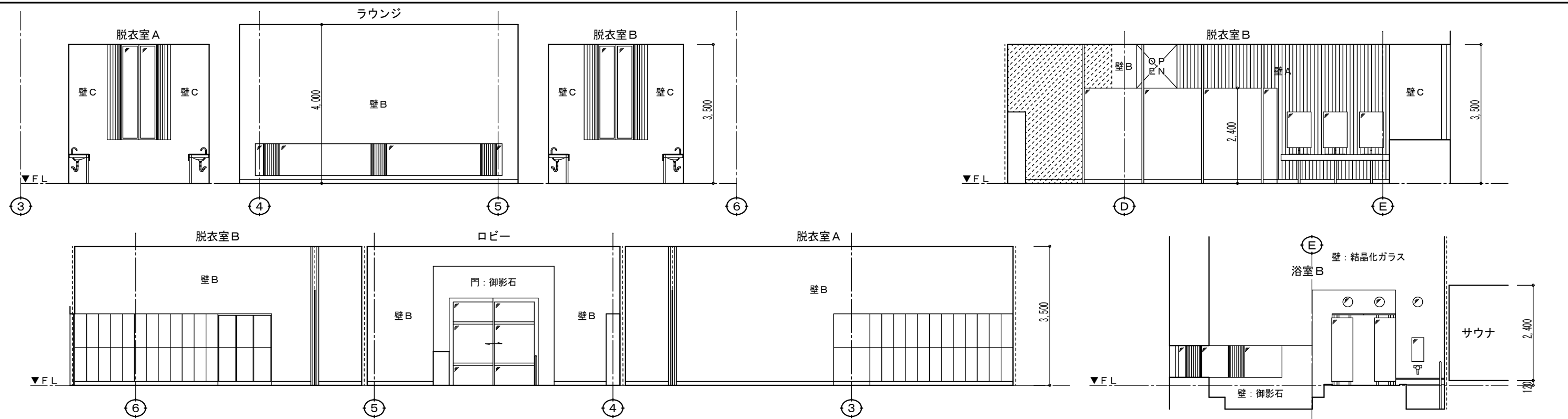
さかいポートサウナ 【既存】平面図(4 F)・展開図
