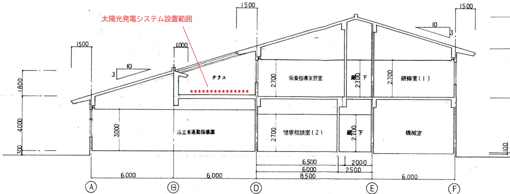
B-1 断面図 1:100
